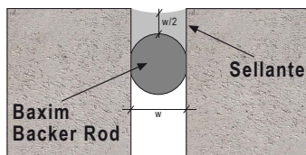
JUNTA DE EXPANSION
